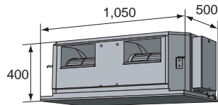
ARXC36LATH : 45kg (unit: mm)
